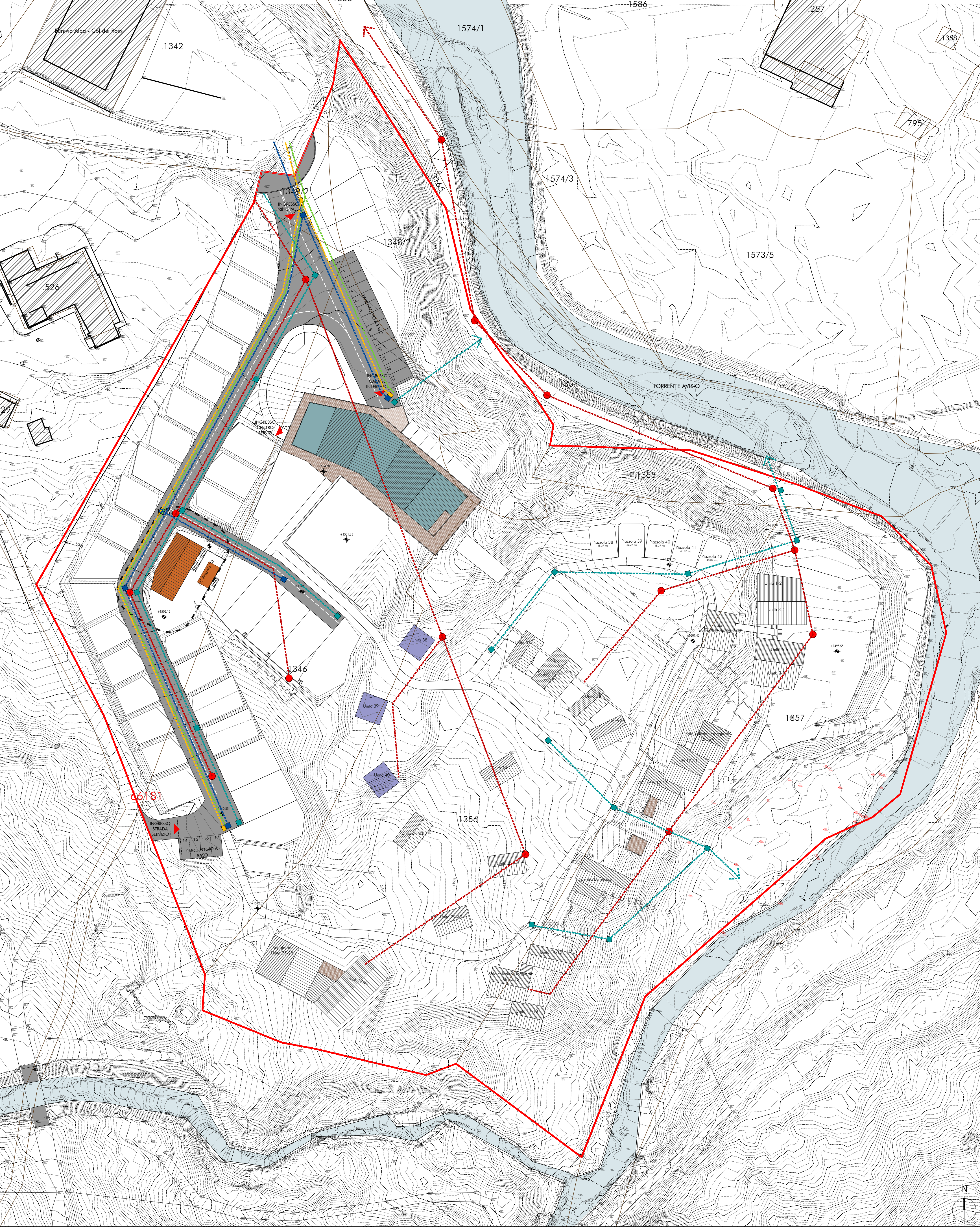
PLANIMETRIA scala 1:500
